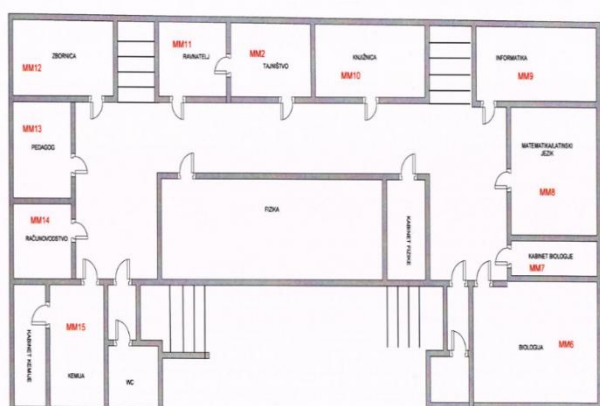
GINNAZIJA NOVA GRADIŠKA prizemlje
