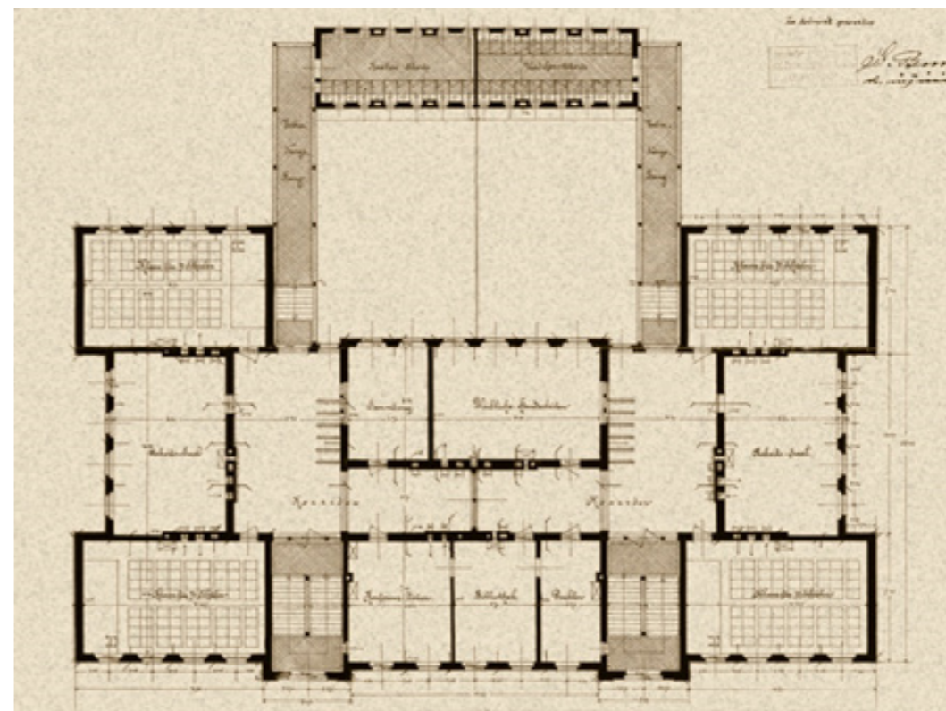
Tlocrt prizemlja
