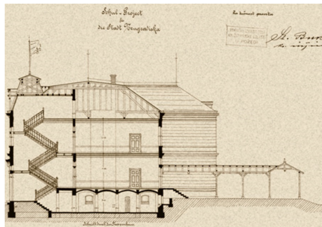
Presjek
